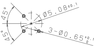
プリント板推奨加工図
