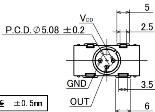
底面図
